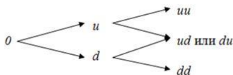
Рисунок 2. Состояния рынка для трех периодов (дат)
