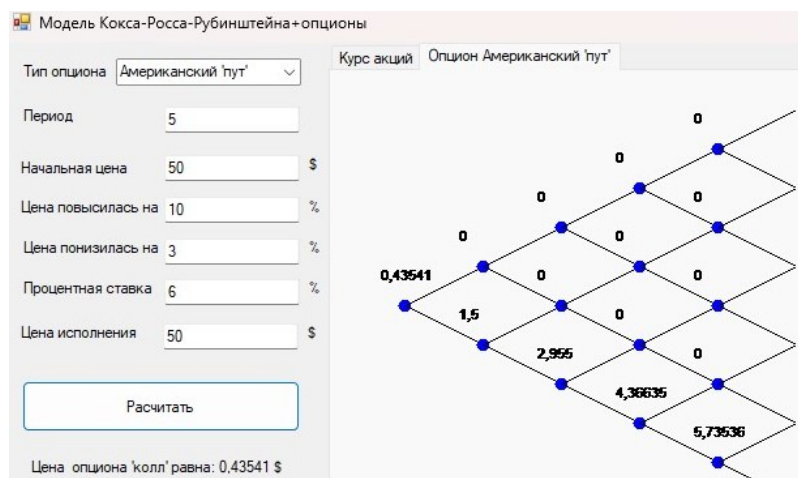
Рисунок 5. Цена американского опциона "пут"
