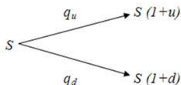
Рисунок 1. Биномиальное дерево для двух периодов
