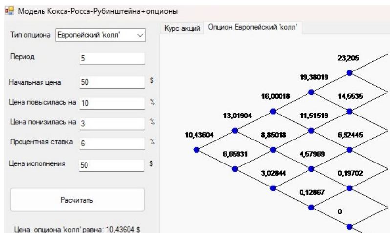
Рисунок 4. Цена европейского опциона "колл"
